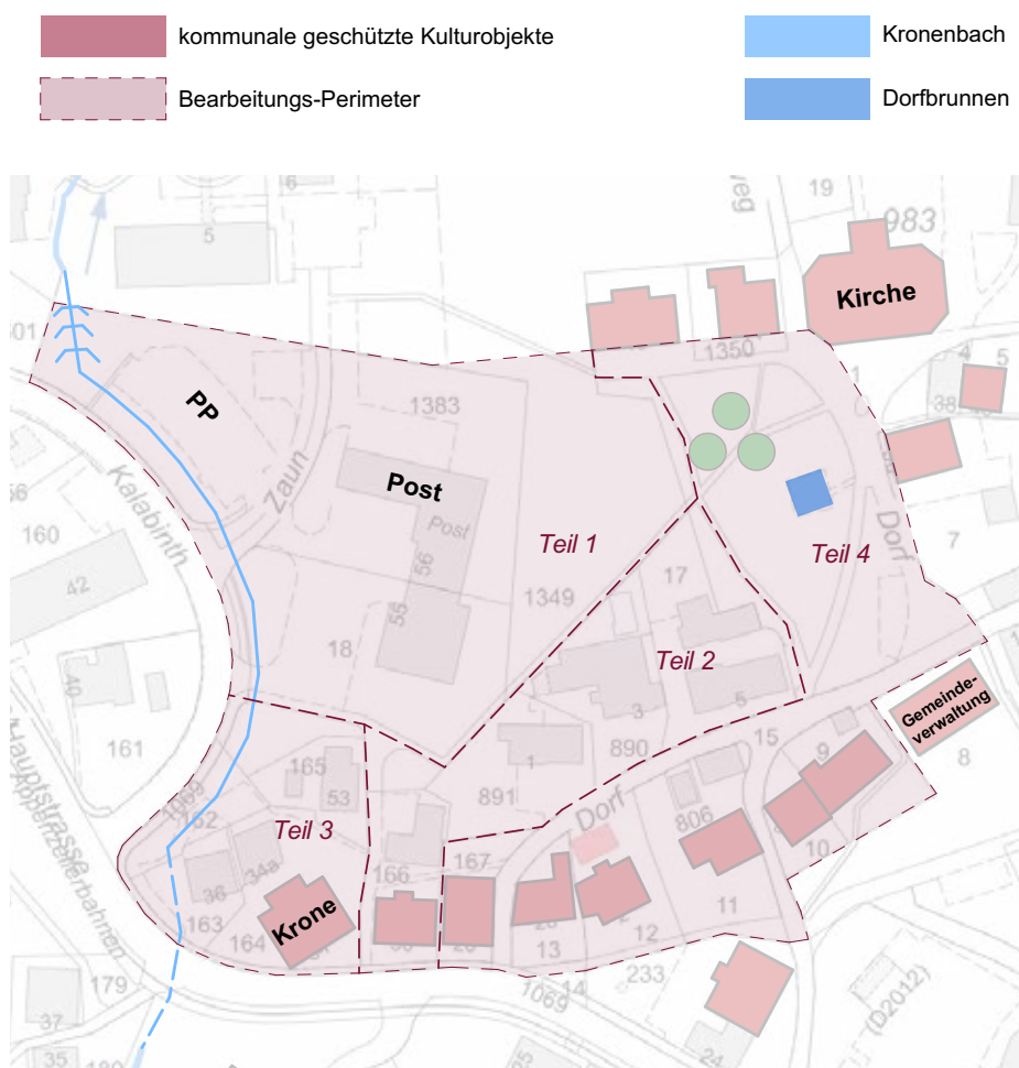
Planungsperimeter Dorf/Hinterdorf mit Teilgebieten
